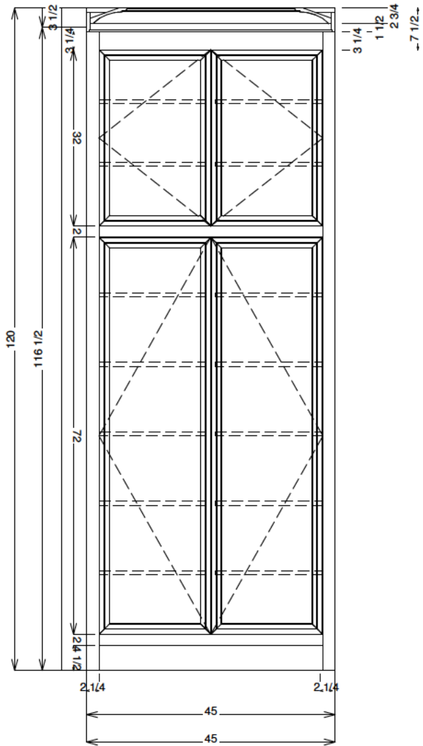
6.10 3 MASTER VESTIBULE ELEVATION Scale: 1/2" = 1'
